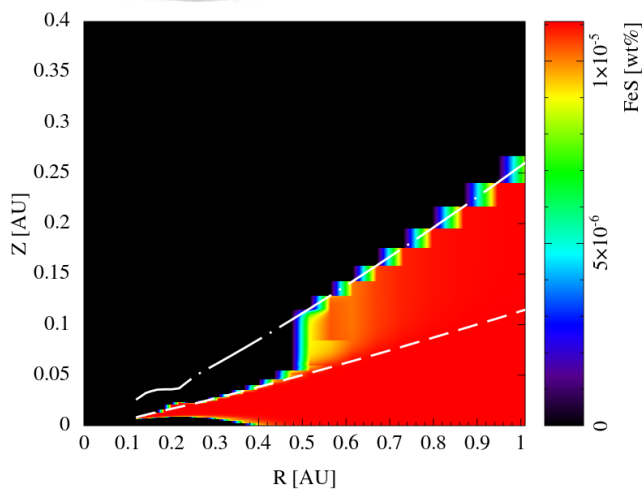
Fig.1 : Les scientifiques ont calculé la composition chimique de la poussière dans la nébuleuse qui entourait le Soleil jeune. Ici : la répartition de sulfure (avec à gauche le soleil jeune). Crédits : Francesco Pignatale.
